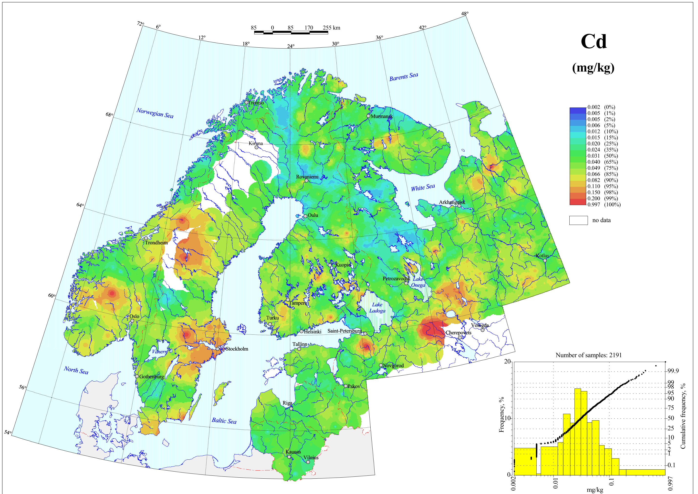
Cadmium in C-horizon, Grain Size <2 mm, Aqua regia Extraction
